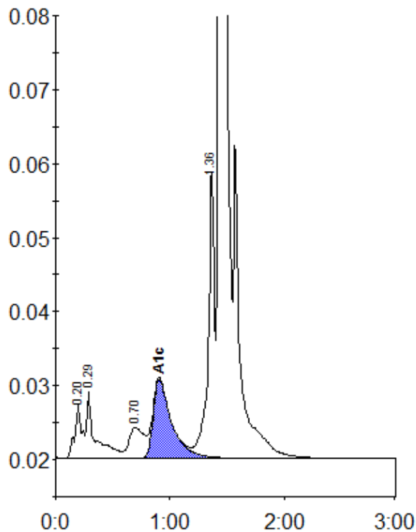
Peak table - ID: 10465811
